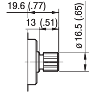
DIN 5482 B17x14
